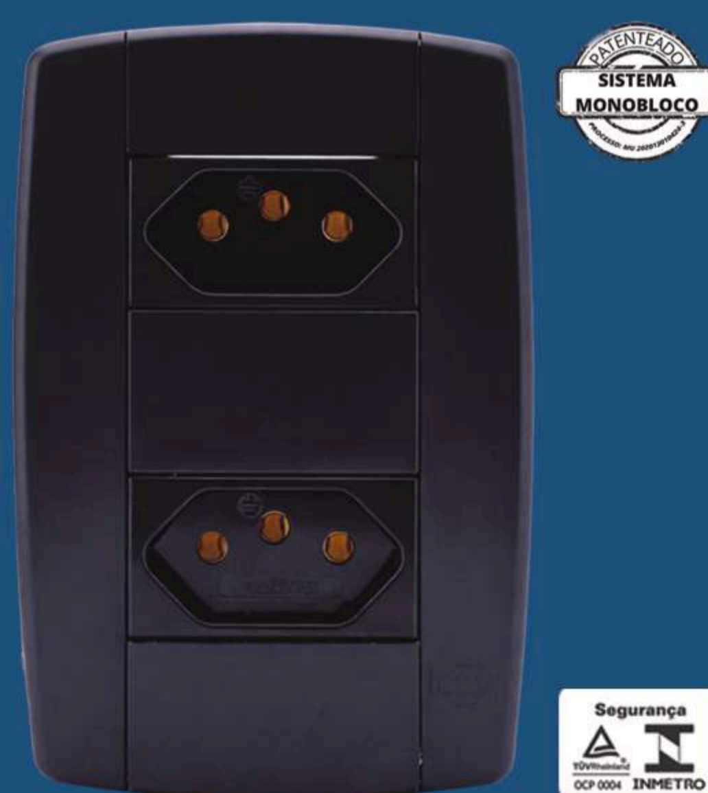
CJ. 2 Tomadas Monobloco 10A 250V - Cód. 871204 Inner: 15 Master: 180 20A 250V - Cód. 871214 Inner: 15 Master: 180
