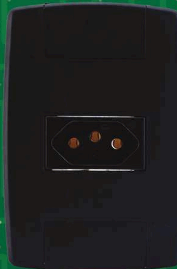
CJ. 1 Tomada 10A 250V - Cód. 871404 Inner: 20 Master: 240 20A 250V - Cód. 871414 Inner: 20 Master: 240
