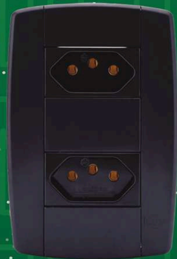
CJ. 2 Tomadas Monobloco 10A 250V - Cód. 871204 Inner: 15 Master: 180 20A 250V - Cód. 871214 Inner: 15 Master: 180
