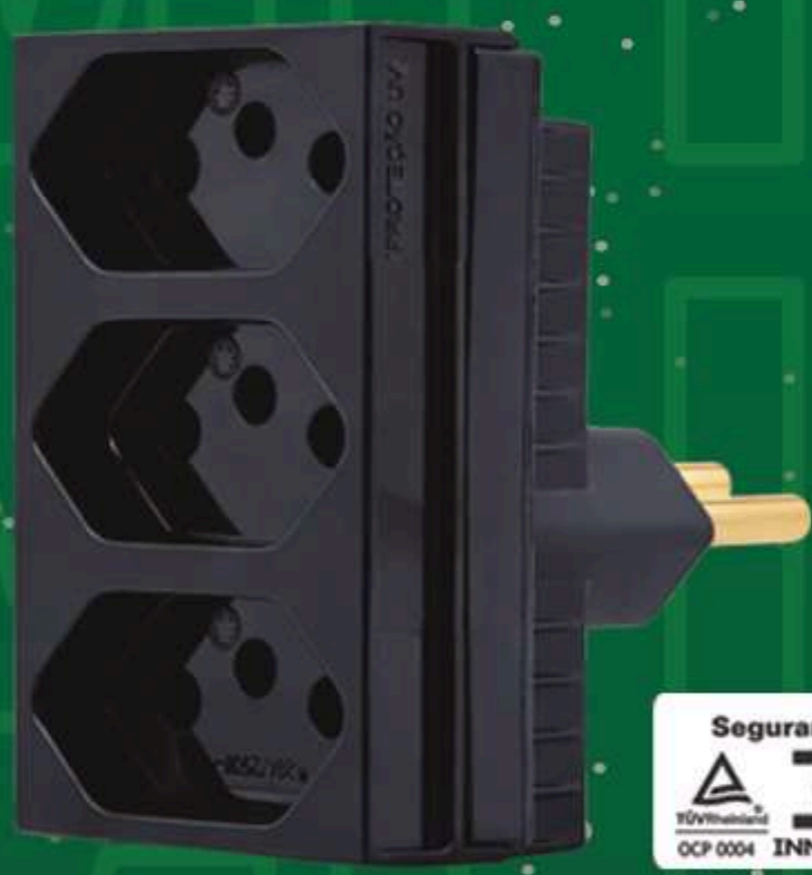
Pino Adaptador 3 Saídas Monobloco 2P+T 20A 250V~ Preto Cód. 12320 Inner: 10 Master: 100
