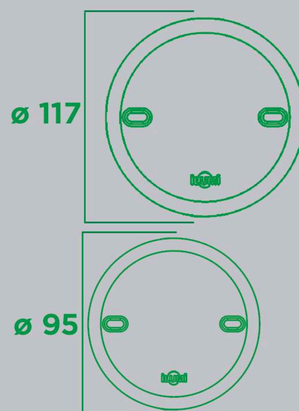
Placa Cega Redonda 3" PT Cód. 20442
