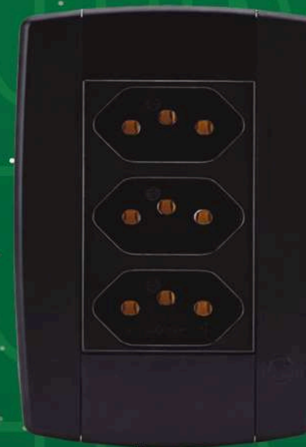
CJ. 3 Tomadas Monobloco 10A 250V- Cód. 871234 Inner: 10 Master: 100 20A 250V - Cód. 871244 Inner: 10 Master: 100
