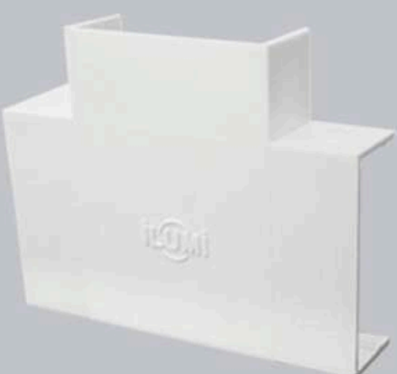
Tipo T 40x16: Cód. 62040 Inner: 30 Master: 360 50x20: Cód. 62041 Inner: 25 Master: 300
